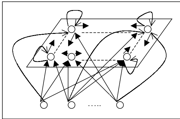
Figura 3.1. Estructura de un mapa de Kohonen.
