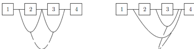
Figura 1. Ejemplo vine regular y no regular para cuatro variables
