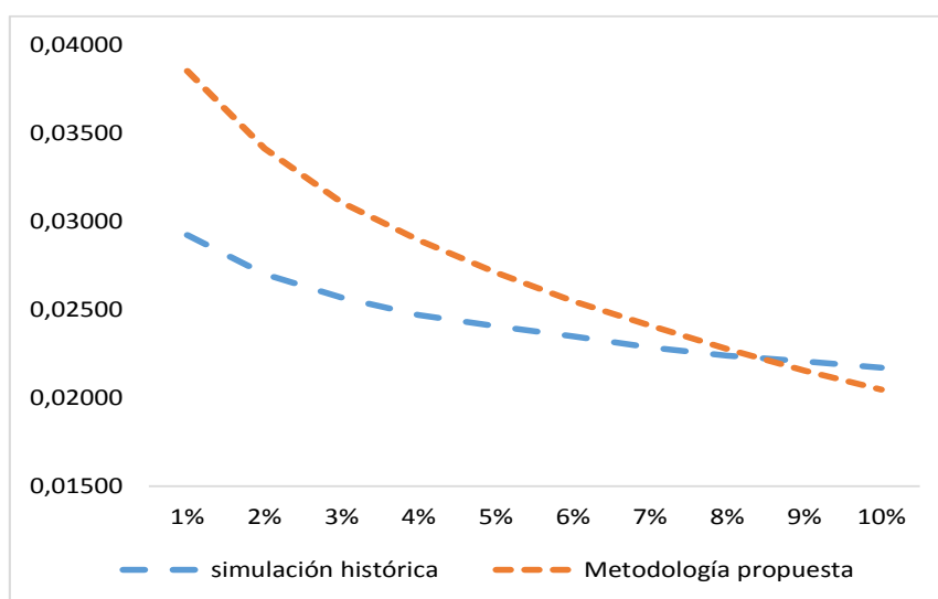
Figura 9. Comparación VaR para el portafolio por ambos métodos.
