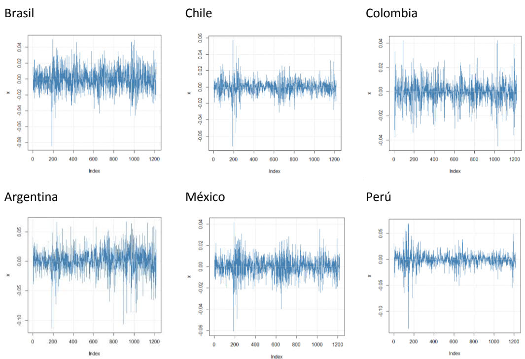
Figura 5. Series de los log retornos diarios
