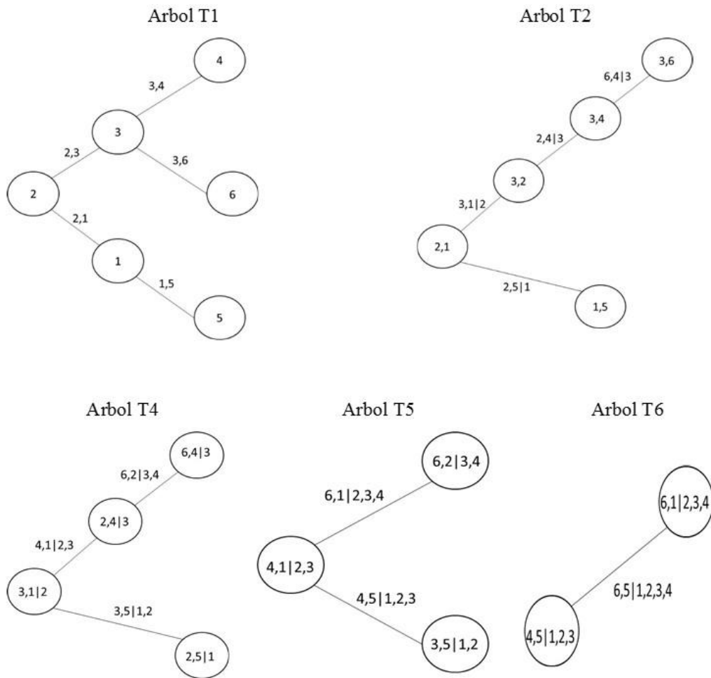
Figura 8. R-vine estimada. Los números indican el índice de los 6 mercados como sigue: 1=BR, 2=MX, 3=CH, 4=COL, 5=ARG, 6=PER
