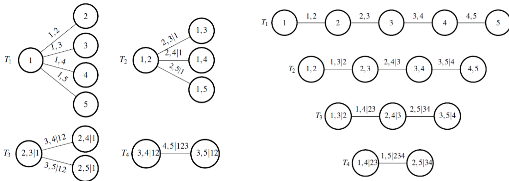
Figura 3. A la izquierda ejemplo C-vine, derecha D-vine con cinco variables
