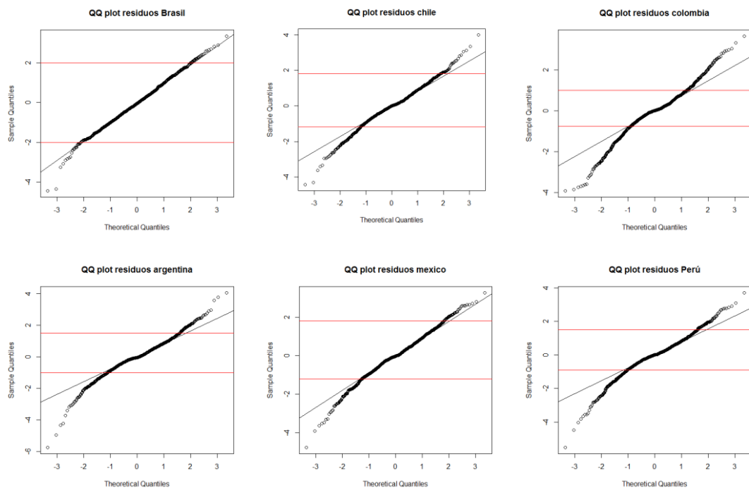
Figura 7. QQ plots para residuales estandarizados y umbrales de estimación para colas PG
