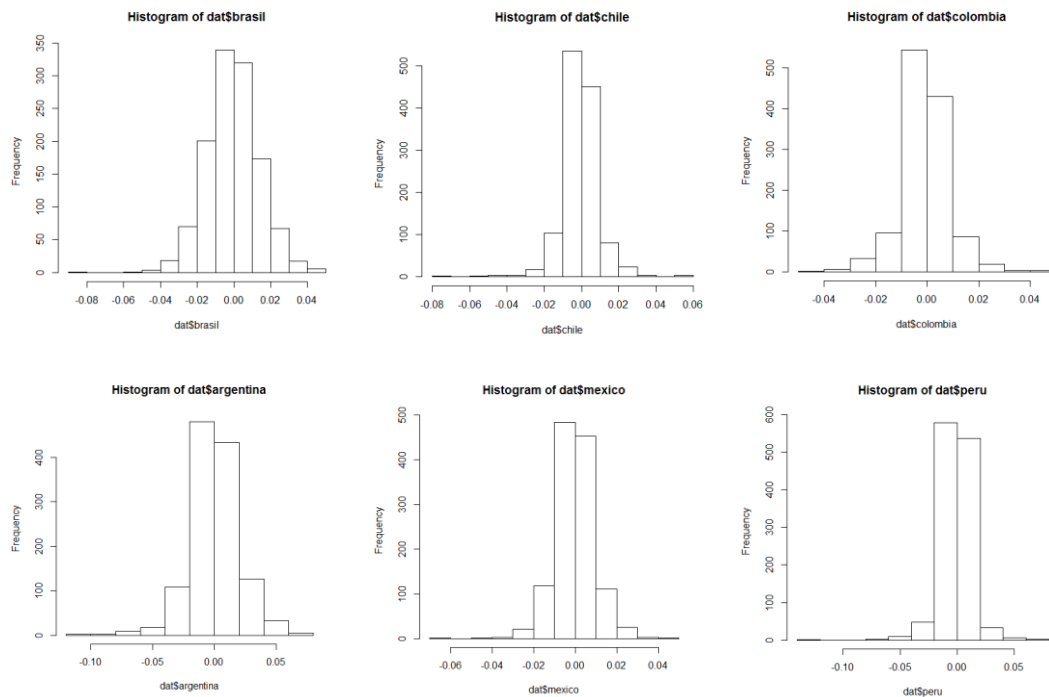
Figura 4. Histograma de los log retornos
