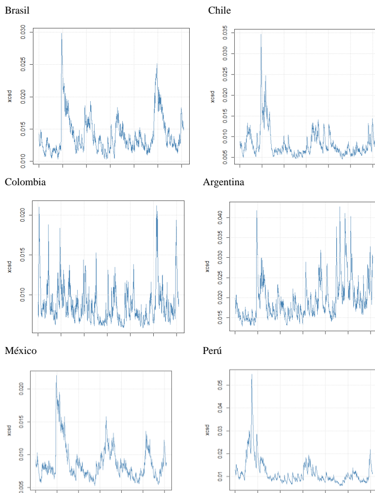
Figura 6. Estimación de volatilidad condicionada para los seis retornos en el periodo nov-2011 a oct-2015
