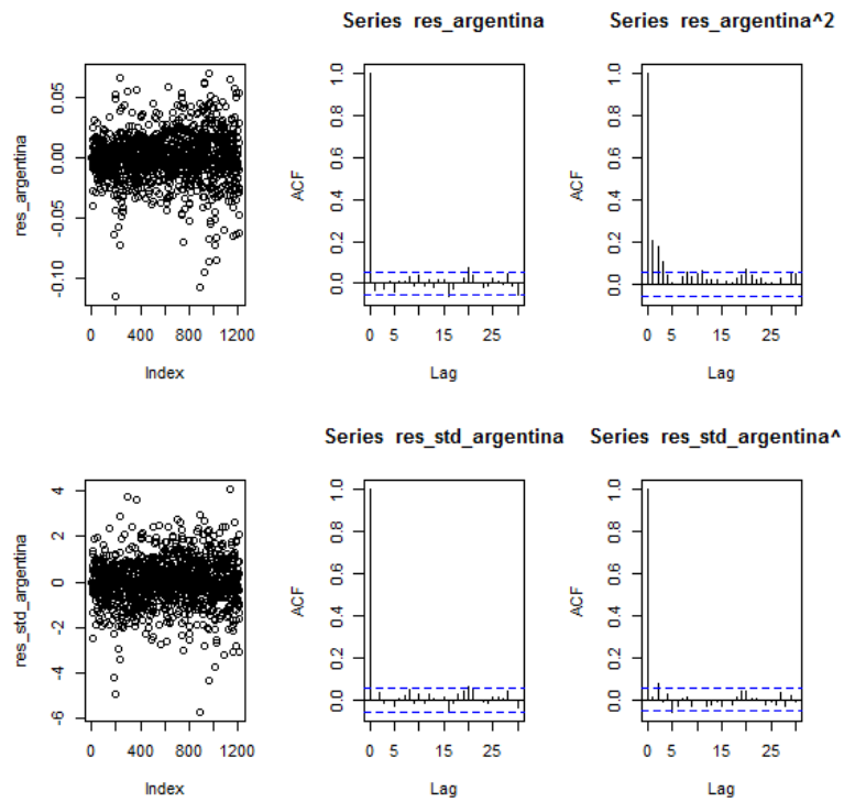
Figura A4. Autocorrelogramas simples y parciales para los residuales y residuales 2 índice Argentina
