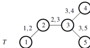
Figura 2. Ejemplo de árbol: N = \{1,2,3,4,5\} , E = \{\{1,2\}, \{2,3\}, \{3,4\}, \{3,5\}\}
